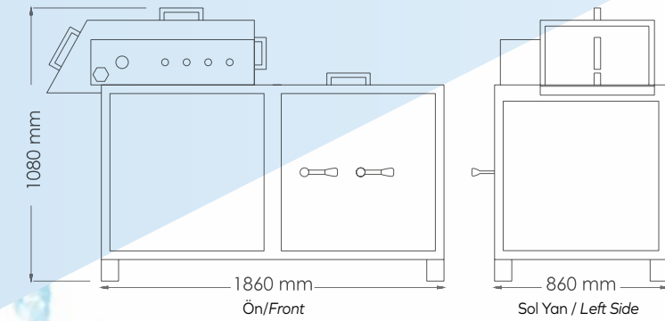
Genel Ölçüler / General Dimensions
